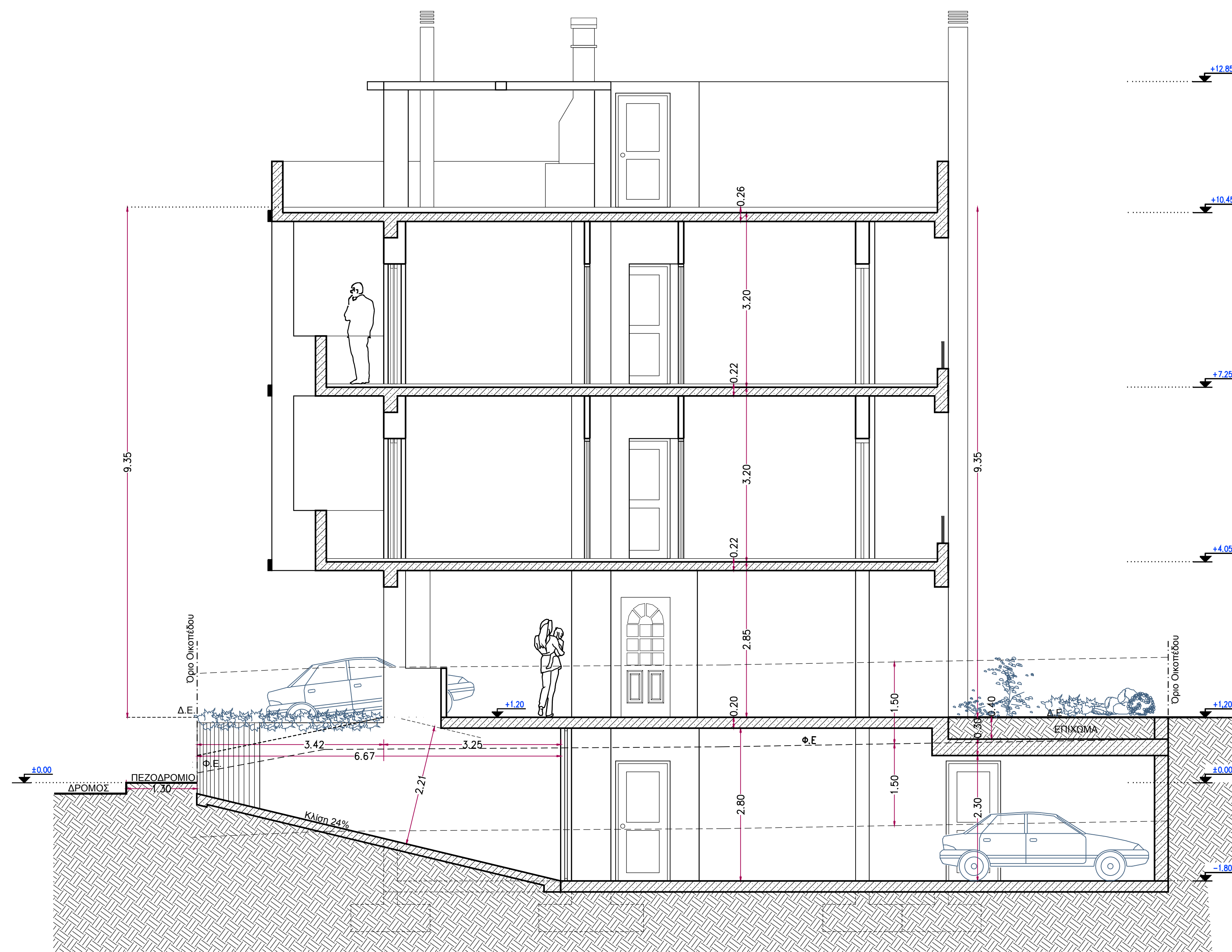
ΤΟΜΗ Α-Α
