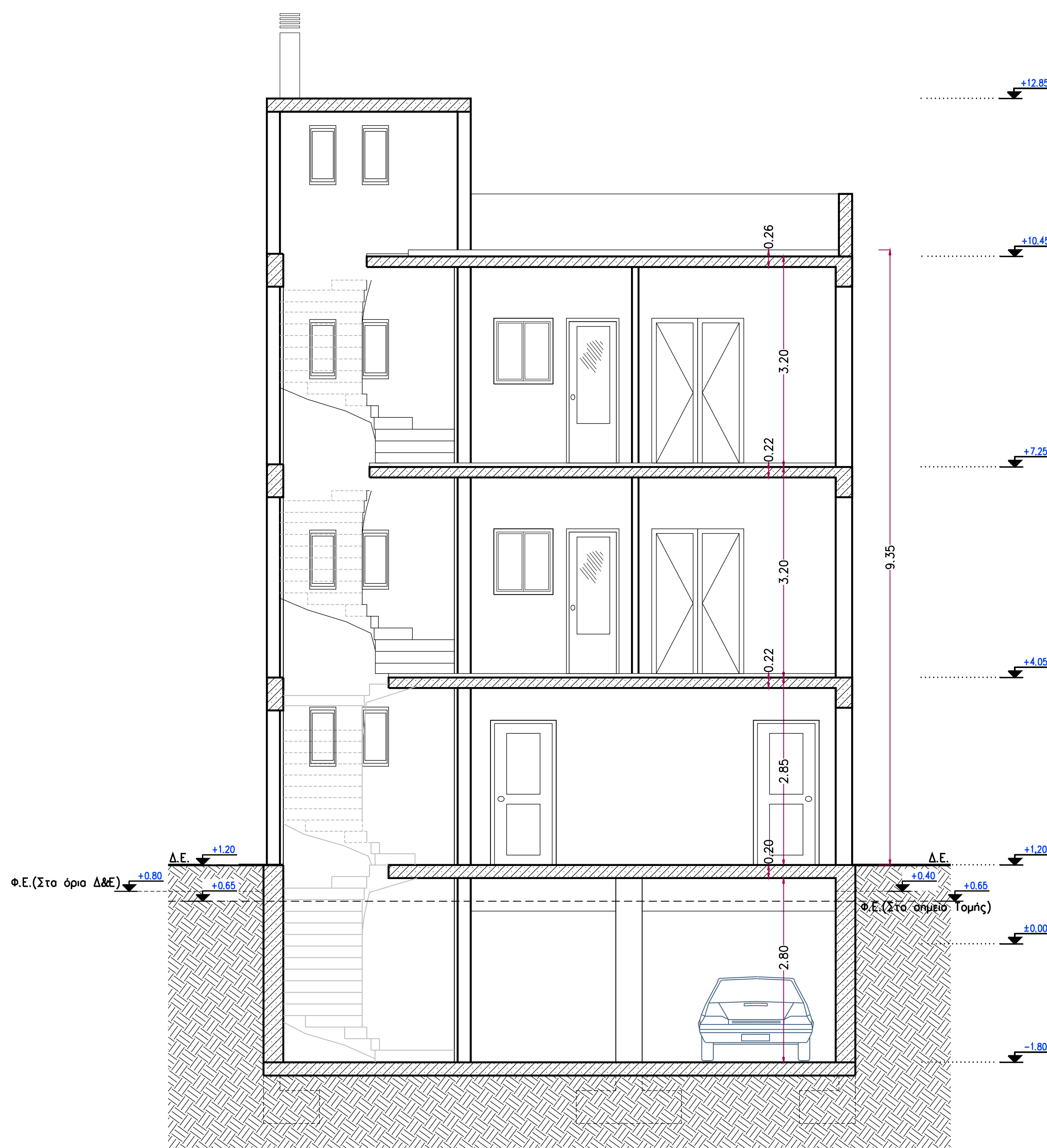
ΤΟΜΗ Β-Β
