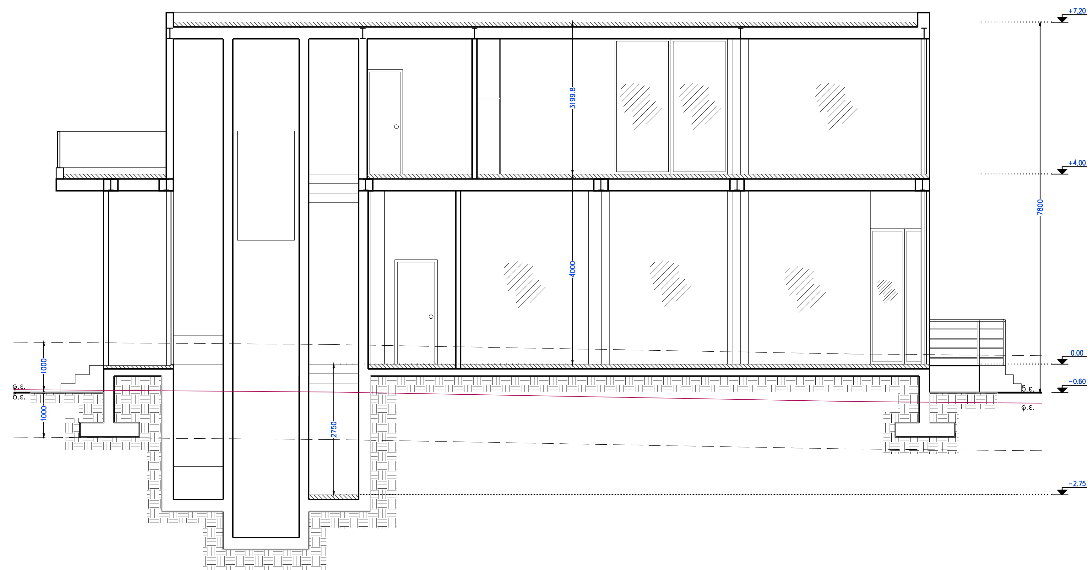
ΤΟΜΗ Β-Β
